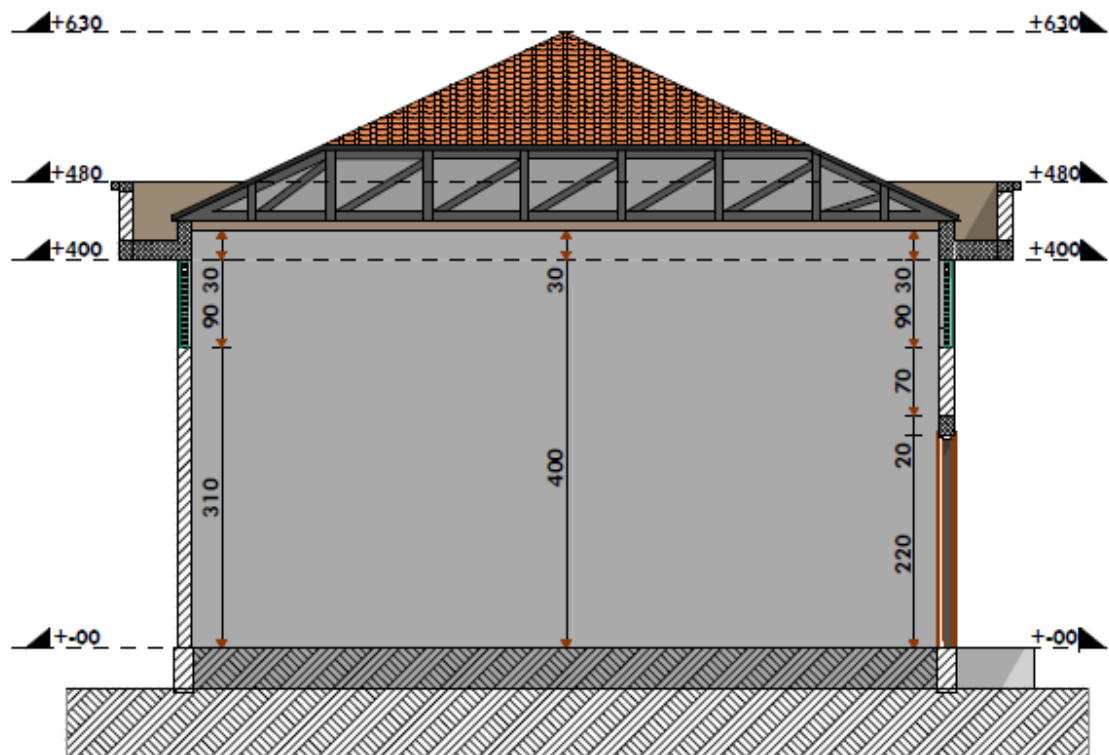
COUPE AA - SECTION AA
