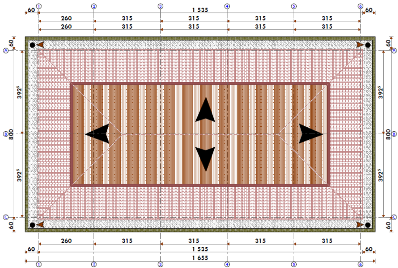
PLAN DE TOITURE - ROOF PLAN
